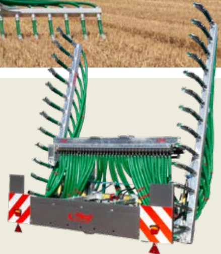
Abb. Transportschutz mit Beleuchtung und Warntafel
