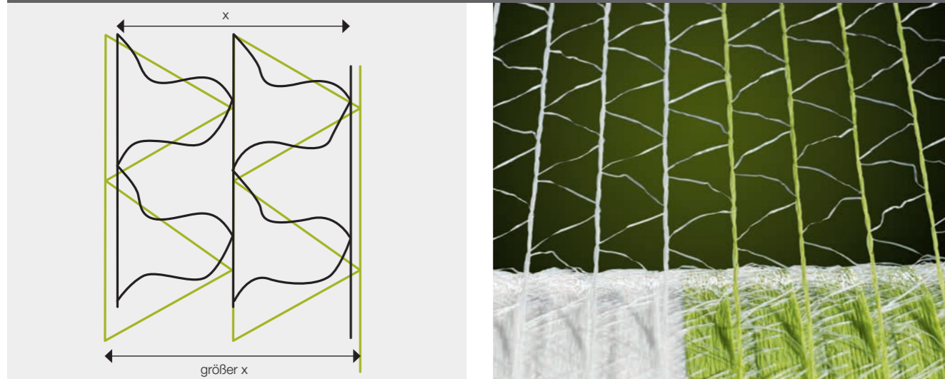
CLAAS ROLLATEX Netz: Schussfäden mit Längenreserven
