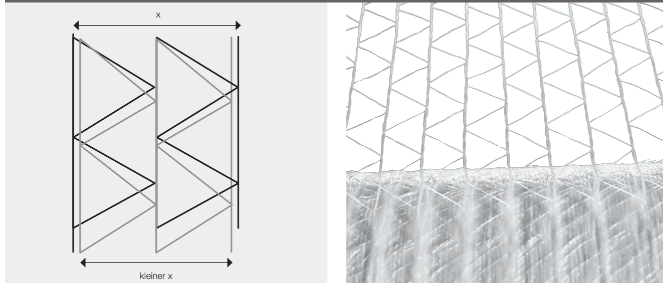
Standardnetz ohne Längenreserven
