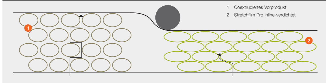
Folienverdichtung Pre-Stretch-Verfahren
