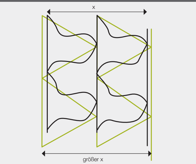
CLAAS ROLLATEX Netz: Schussfäden mit Längenreserven
