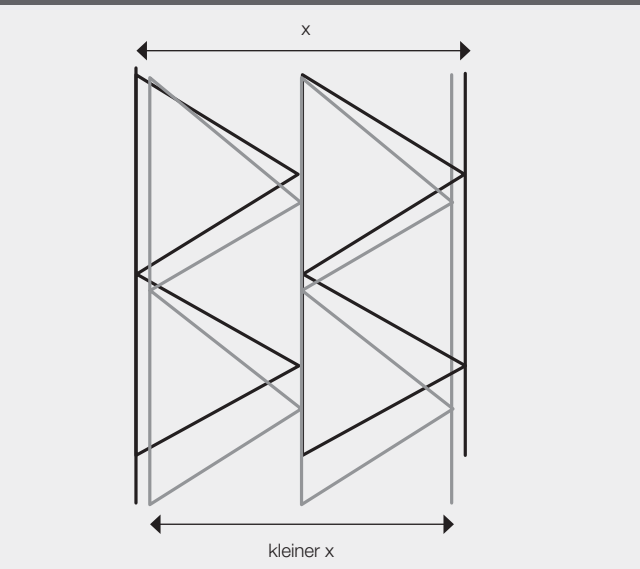
Standardnetz ohne Längenreserven
