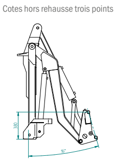
Cotes hors rehausse trois points
