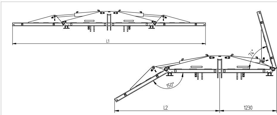
Largeur de déblayage réglable en continu par les 2 panneaux latéraux, grillage de rehausse (en option)
