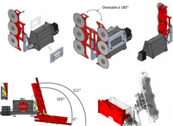
Montage à gauche sur chargeur télescopique
