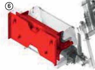
Limiteur de charge comme adaptateur d'amortissement : si la pression d'appui est trop élevée, la tête bascule en arrière pour assurer la protection en cas de blocage des lames de scie.
