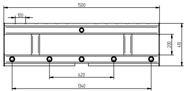
Illustration avec arceau de sécurité qui assure la protection anti-glissement, par ex. pour les tas de bois, balles, profils en acier, etc. Installation a posteriori rapide et facile !
