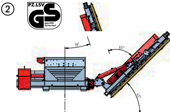
Certification GS : dispositif d'inclinaison 45° - Le modèle testé est conforme aux exigences mentionnées dans la loi allemande sur la sécurité des produits (ProdSG) ainsi qu'au niveau d'expérience actuel en matière de prévention des accidents.
