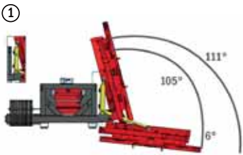
Dispositif d'inclinaison à 111° - pour coupes verticales et horizontales. L'angle peut alors être ajusté en continu.
