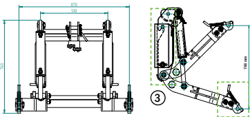
Relevage avant 1,8 t
