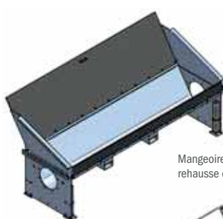
Mangeoire d'accueil avec montage latéral de tuyau
