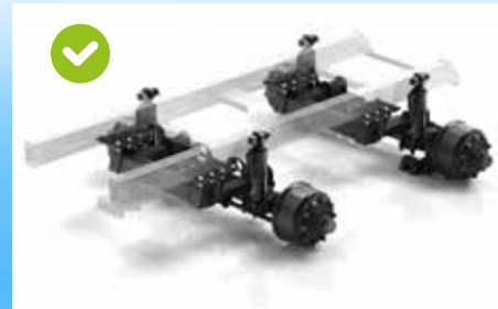
Train de roues à suspension hydraulique
